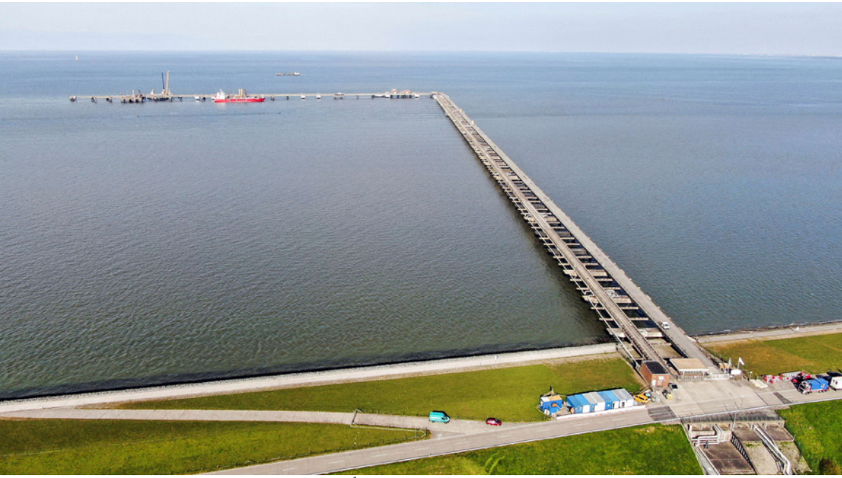
صورة جوية لنصبة قيد الإنشاء مخصصة لاستقبال حمالات الغاز المسال في ميناء فيلهمشافل في شمال ألمانيا
